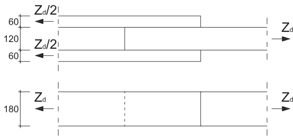
Abbildung 111: Zugstoß
